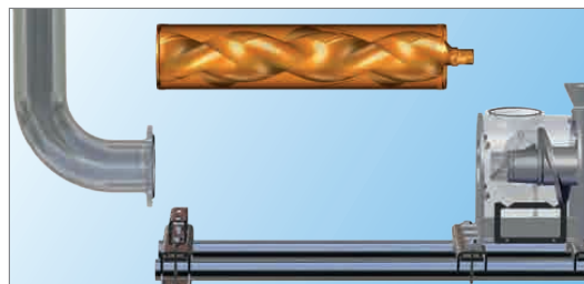
Schritt 3: Stator und Rotor nach vorne bewegen und aus dem Gehäuse herausziehen.
