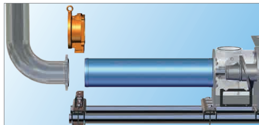
Schritt 2: Zugstangen druckstutzenseitig lösen, Druckstutzen nach oben entnehmen.
