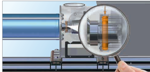
Schritt 1: Verschlusschrauben lösen und Verbindungsbolzen entfernen.
